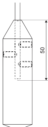
Obr. 19: Náčrt závaží lanové elektrody
