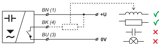
Obr. 14: Zapojení snímače s výstupem typu NPN (provedení N, NT, Xd)
