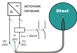
подключение датчика к катушке реле
