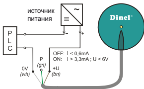
подключение датчика к логическому устройству ПЛК
