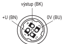
Obr. 9: Vnitřní pohled na konektorovou zásuvku (typ ELWIKA, ELKA)
