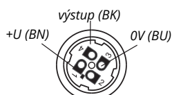
Vnitřní pohled na konektor
