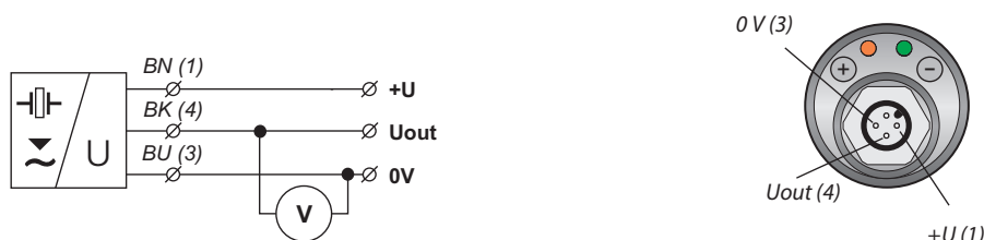
Obr. 6: Připojovací schéma a vnitřní pohled na konektor hladinoměru DLM (varianta - U)
