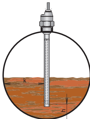
Obr. 3: Instalace hladinoměru s referenční trubkou
