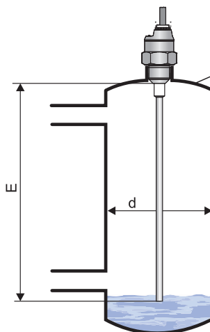
Obr. 1: Instalace hladinoměřů s tyčovou elektrodou
