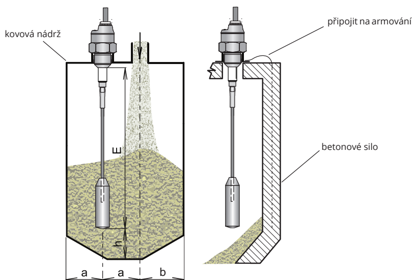
Obr. 4: Instalace hladinoměrů s lanovou elektrodou
