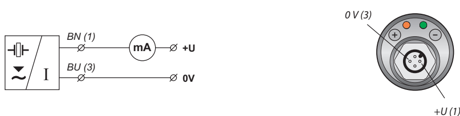
Obr. 5: Připojovací schéma a vnitřní pohled na konektor hladinoměru DLM (varianta - I)
