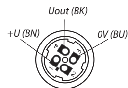
Obr. 7: Vnitřní pohled na konektorovou zásuvku (varianta "C")
