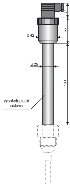
vysokoteplotní provedení CLM-36_T
