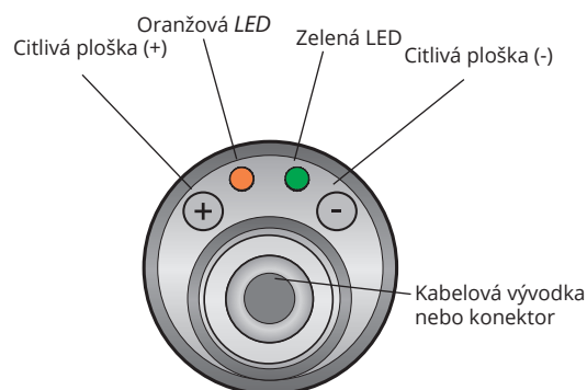
Obr. 15: Pohled shora na snímač
