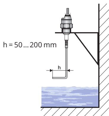
Obr. 6: Ohnutí konce elektrody při snímání neznámých kapalin
