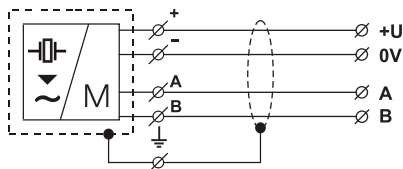
Рис. 16: Схема присоединения измерителя уровня с протоколом Modbus ULM-70_--_M
