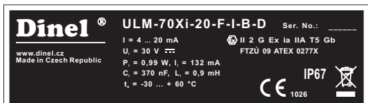
Пример таблички для оборудования типа ULM-70Xi-20-F-I-B-D
