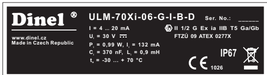
Пример таблички для оборудования типа ULM-70Xi-06-G-I-B-D
