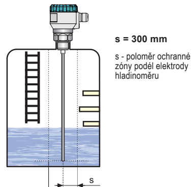
Obr. 12: Instalace hladinoměru mimo překážky v nádrži
