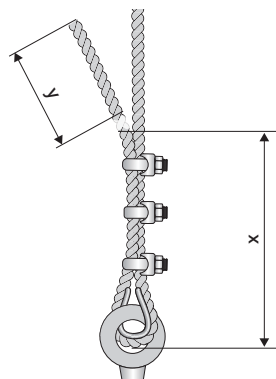
Obr. 30b: Náčres zakončení lana pro typ 36, 37
