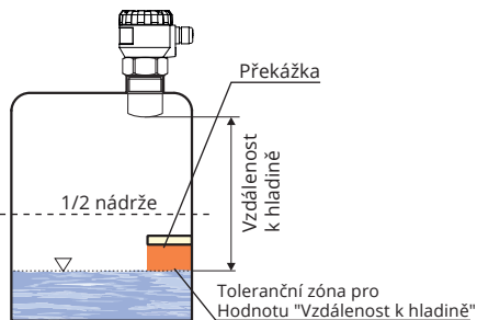
Obr. 15: Úrovňová vzdálenostní zóna "Nastavení vzdálenosti hladiny"
