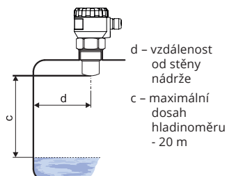
Obr. 3: Vzdálenost hladinoměru od stěny nádrže
