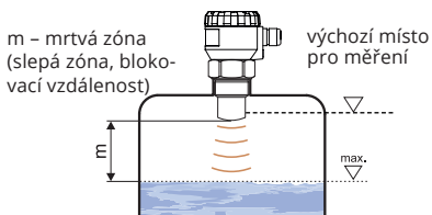
Obr. 2: Mrtvá zóna hladinoměru
