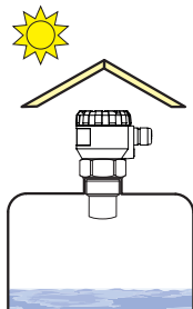
Obr. 11: Stínící kryt proti přímému slunečnímu záření
