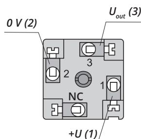
Vnitřní pohled na konektorovou zásuvku variantu "G"
