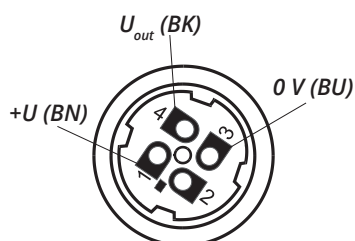
Vnitřní pohled na konektorovou zásuvku varianta "C"
