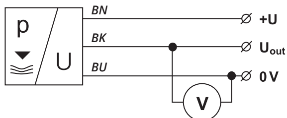
Připojovací schéma snímače PPM-35 pevně připojeným kabelem (varianta U)
