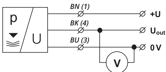
Připojovací schéma a vnitřní pohled na konektor snímače PPM-35 (varianta U)
