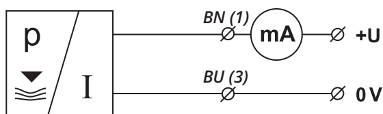
Připojovací schéma a vnitřní pohled na konektor snímače PPM-35 (varianta I)
