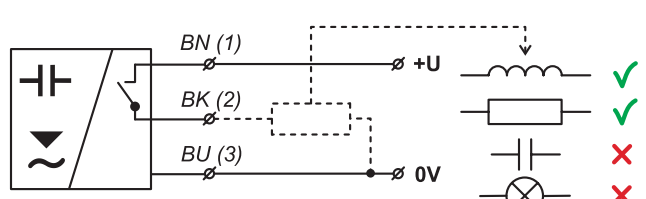
Schéma připojení snímače s typem výstupu „P“ (PNP)
