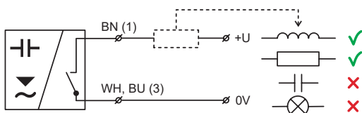
Obr. 7b: Zapojení snímače s výstupem typu „S“ (elektronický spínač) - možná varianta
