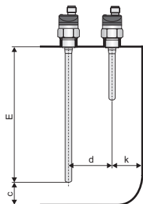
Obr. 1: Svislá instalace snímačů
