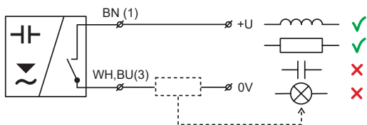
Obr. 7a: Zapojení snímače s výstupem typu „S“ (elektronický spínač) - doporučená varianta
