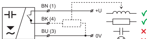
Obr. 8: Zapojení snímače s výstupem typu „P“ (PNP)
