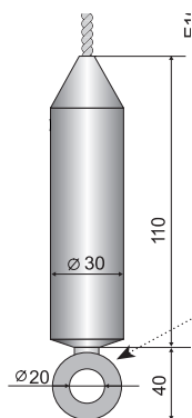
kotvení u varianty GRLM-70_-33 (35)
