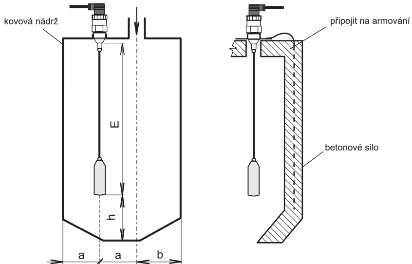
Obr. 3: Instalace hladinoměru s lanovou elektrodou
