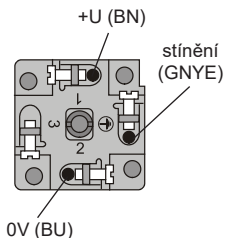
Obr. 7: Vnitřní pohled na konektor s proudovým výstupem
