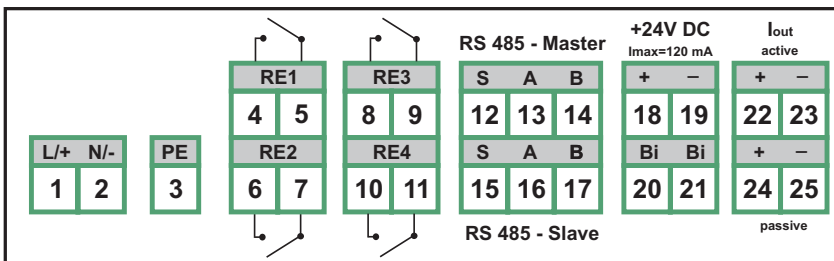
SVORKOVNICE FCU-400-R_-I
