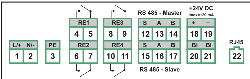
SVORKOVNICE FCU-400-R_-I
